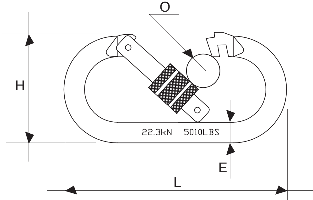
Mousqueton acier à verrouillage par bague à vis. Steel screw gate carabiner
